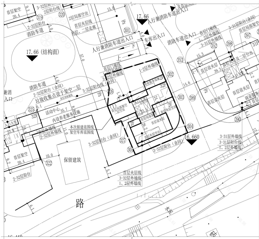
观景阁第1幢总平面图 1:500
